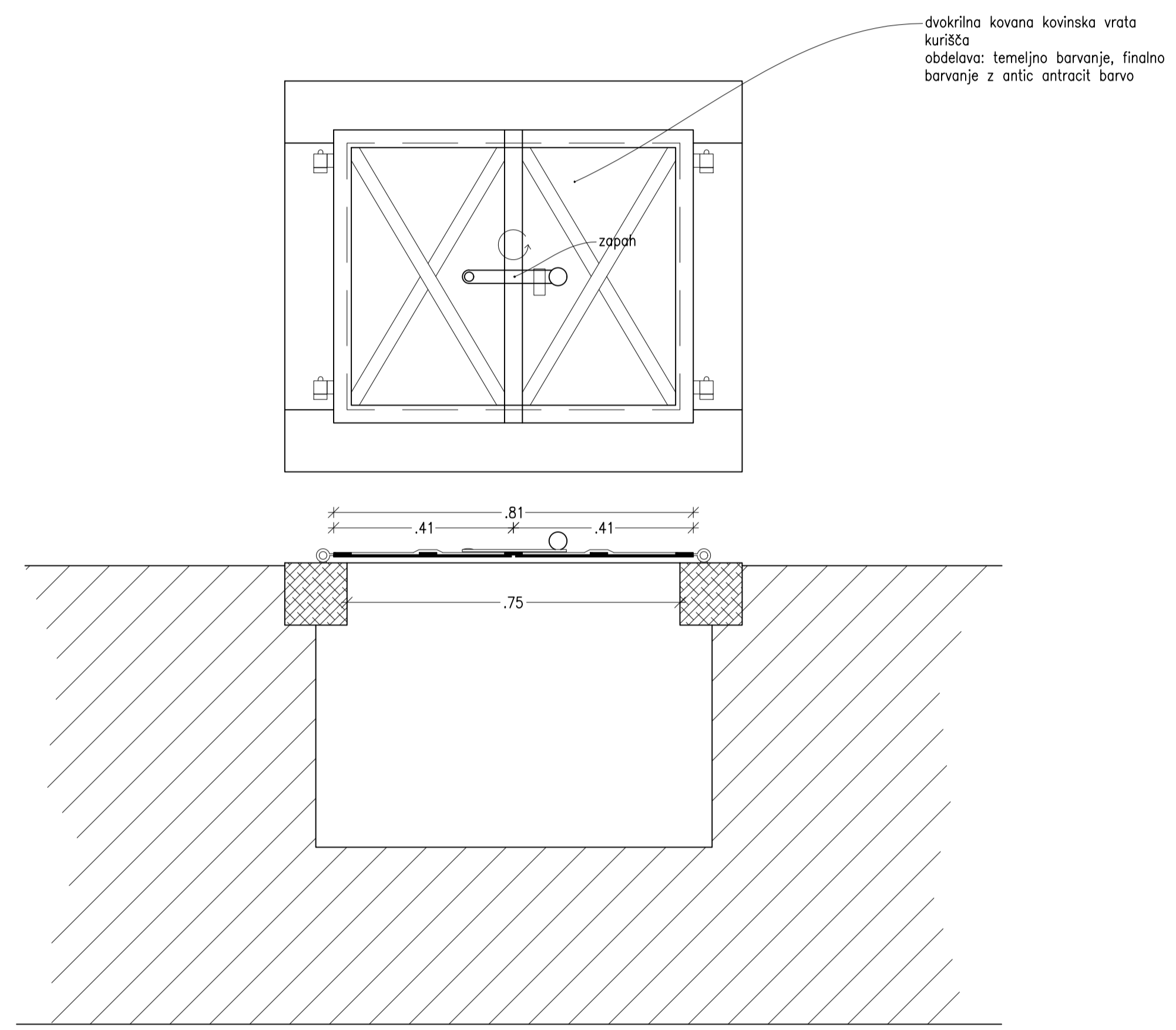
KOVINSKIH VRAT KURIŠČA PRITLIČJE
